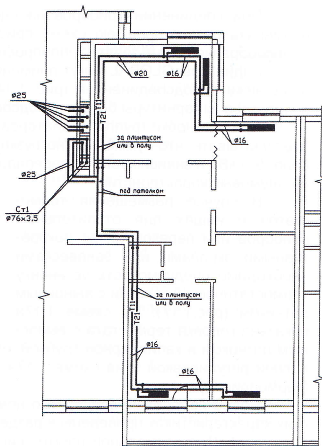
Рис. 1.19. Система отопления с плинтусной разводкой теплопроводов по квартире
