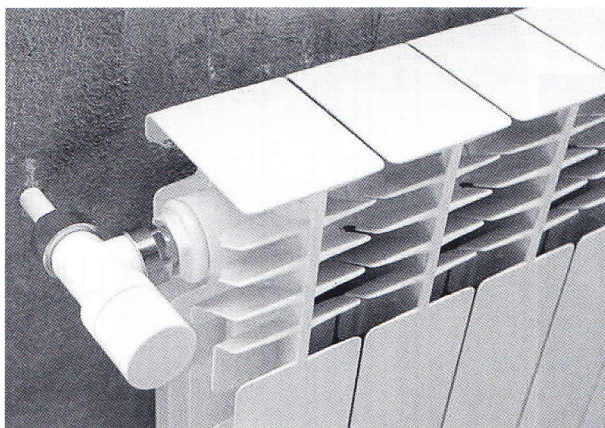
Рис. 1.3. Общий вид (a) и габаритные размеры алюминиевых радиаторов GL: одноколоновых (б) и сдвоенных GL/D (в)
