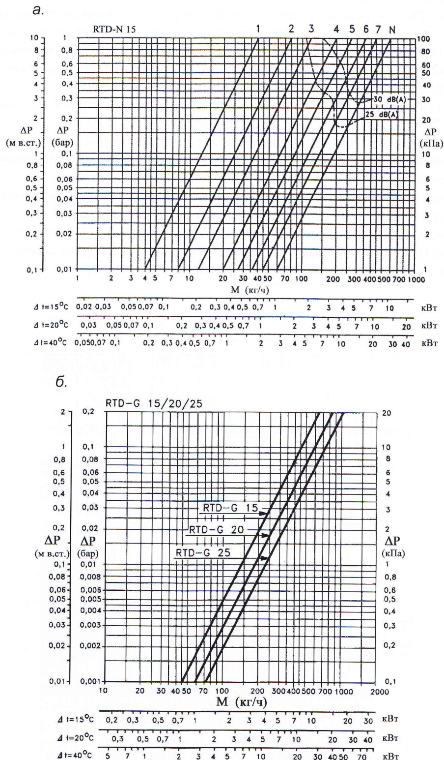
Рис. 2.2. Гидравлические характеристики терморегуляторов фирмы «Данфосс»: а – RTD-N 15 при различных уровнях монтажной настройки клапана для двухтрубных систем отопления с подводками d_y 15 мм; б – RTD-G для гравитационных и насосных однетрубных систем отопления с подводками d_y 15, 20 и 25 мм (при настройке на режим 2К)
